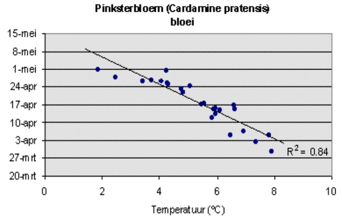
Figuur 2: Bloei van pinksterbloem. De gemiddelde eerste bloeidatum is uitgezet tegen de gemiddelde temperatuur in de periode februari-april. De data omvatten de periode 1947-1968 en 2001-2003
