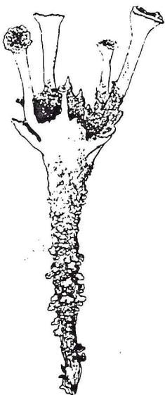
FIG. 1. Cladonia chlorophaea
